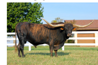
BH ALICE
